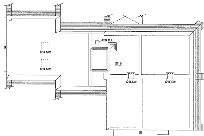
屋上平面図
