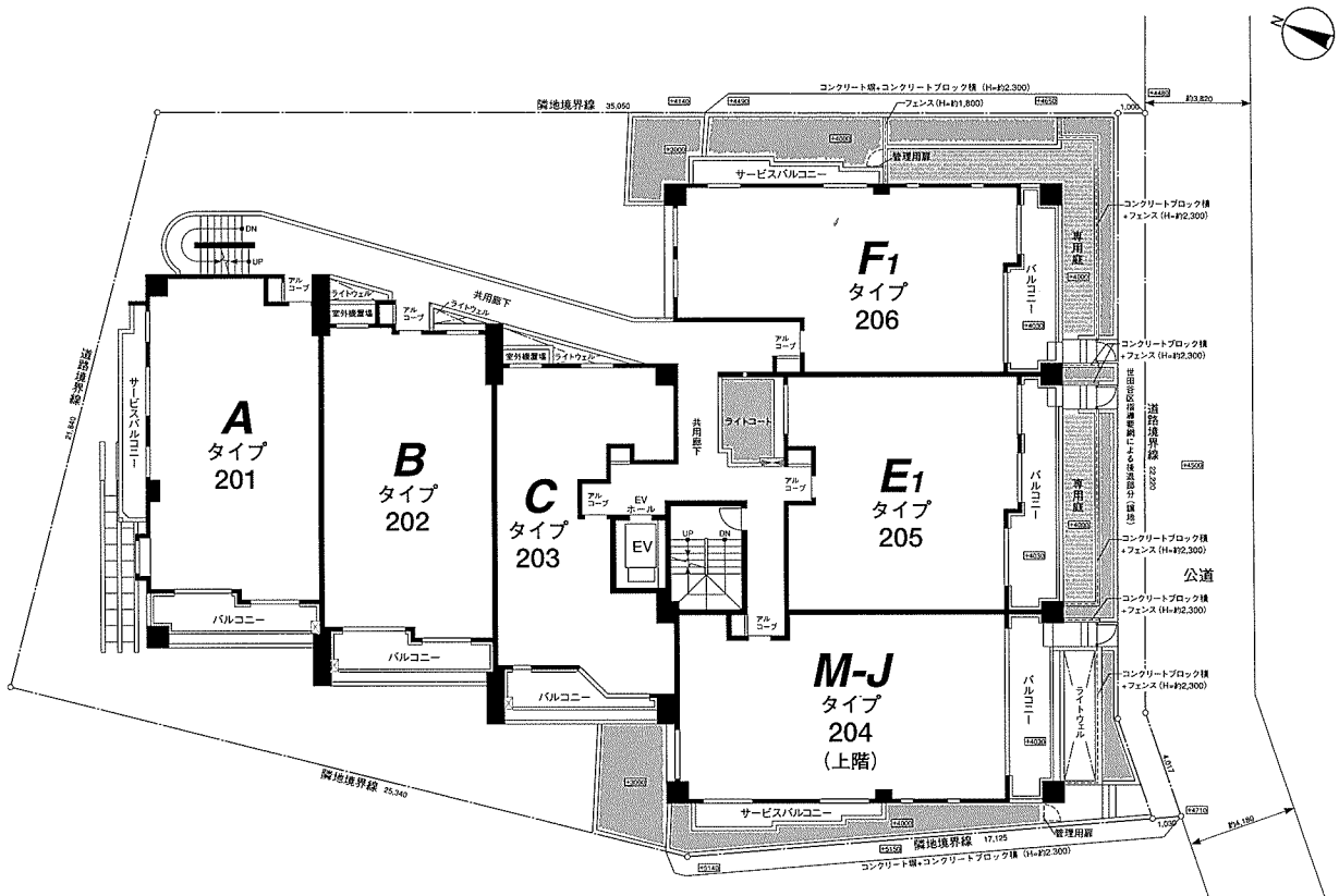
2階平面図
