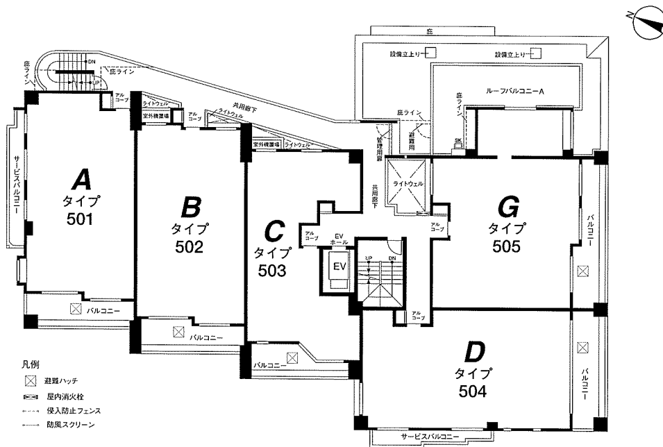
5階平面図
