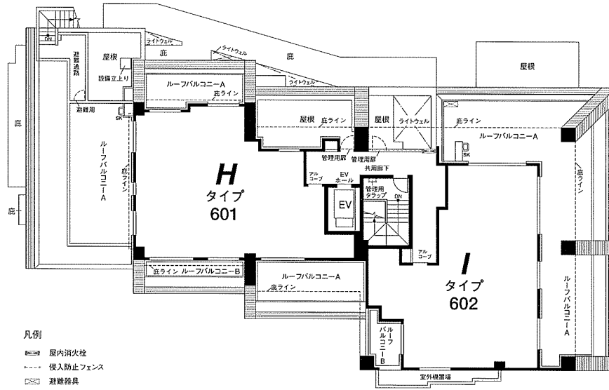
6階平面図
