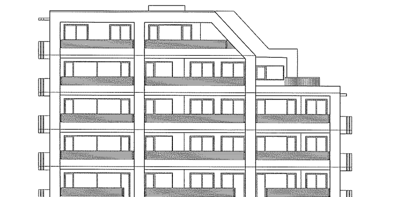
南侧立面图
