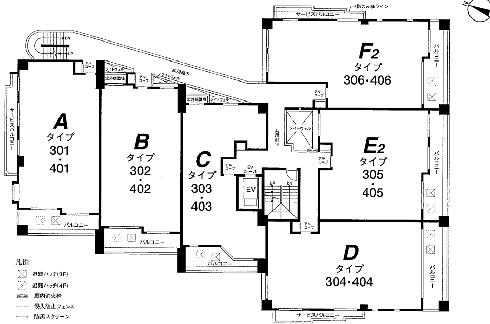
3・4階平面図
