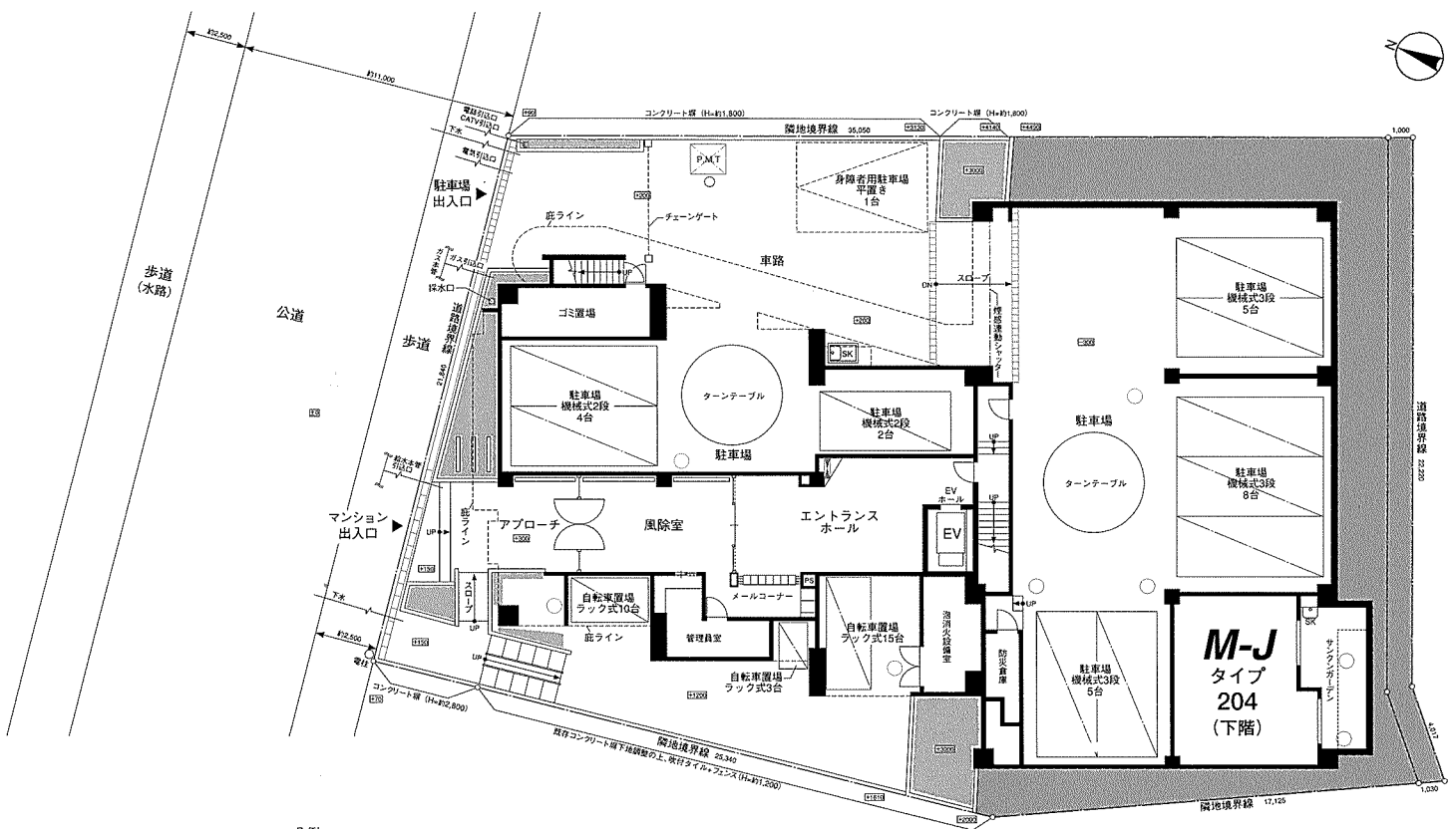
敷地配置図・1階平面図
